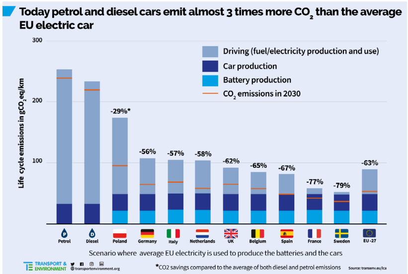
Abbildung 5.1: Aktuelle Diesel- und Benzinfahrzeuge erzeugen fast dreimal so viel CO 2 -Emissionen wie ein vergleichbares E-Auto aus der EU (Quelle: bit.ly/38tVFiN)
