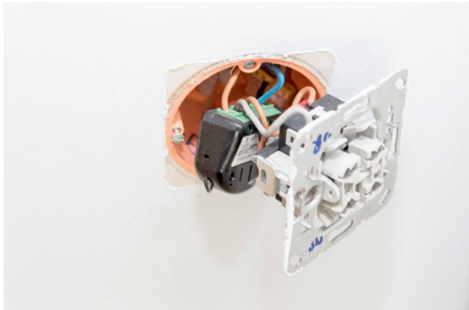
Bild 2.6 Ein Unterputzmodul macht konventionelles Licht smart (© Chris Bertko).
