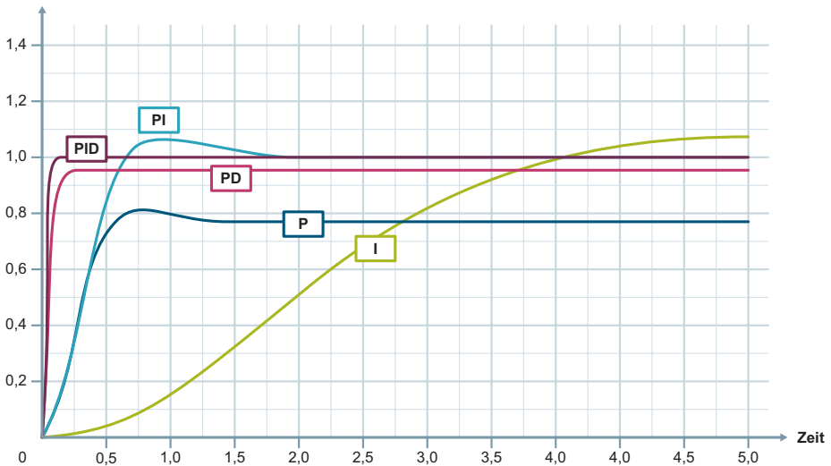
Bild 1.8: Drehzahlregelung; Vergleich des zeitlichen Verhaltens mit verschiedenen Reglertypen. Bei einer sprunghaften Änderung der Eingangsspannung (Sollwert-Sprung) erzeugen die unterschiedlichen Regler das jeweils dargestellte Verhalten der Drehzahl (= Sprungantwort der Regelstrecke).
