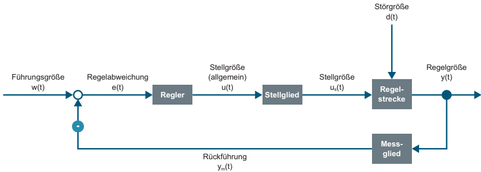
Bild 1.1: Standard-Blockdiagramm. In einem Drehzahl-Regelkreis bedeuten die Bezeichnungen: Führungsgröße = Drehzahl-Sollwert Regelabweichung = Soll-Istwert-Differenz Stellgröße = Sollwert für das Stellglied (Verstärker) Regelstrecke = Servomotor + Mechanik Störgröße = z. B. Belastungsänderungen Regelgröße = Drehzahl Messglied = Drehzahlmessgerät Rückführung = Drehzahl-Istwert
