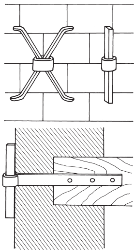
Abb. 4: Balkenanker. Oben Anker-splinte in Kreuz- und Stabform
