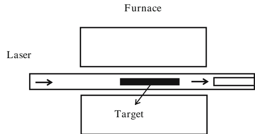
Fig. 2.6 Laser-ablation scheme
