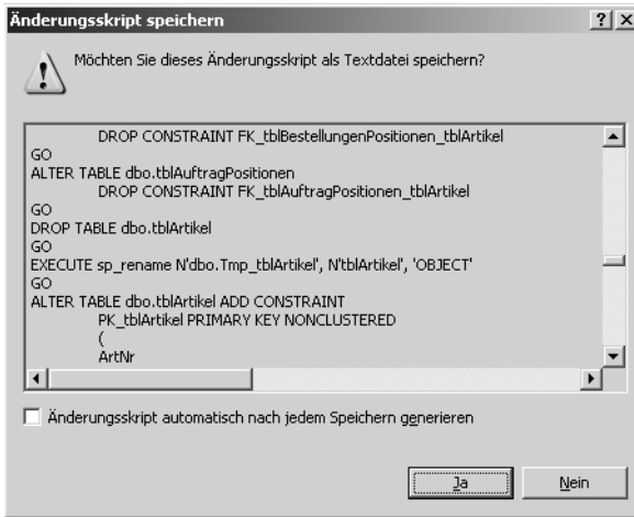
Abbildung 3.44: Änderungsskript
