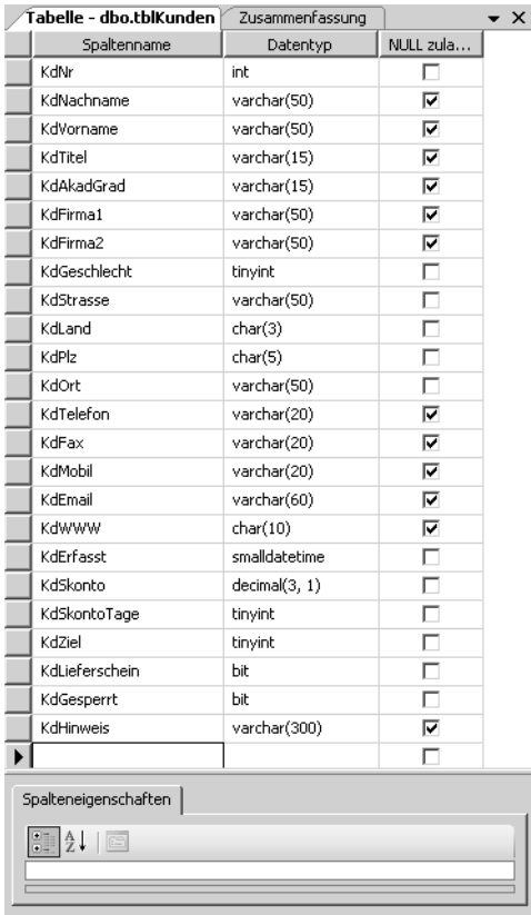
Abbildung 3.15: Kundentabelle
