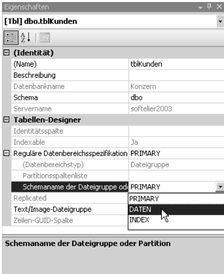
Abbildung 3.42: Tabelleneigenschaften
