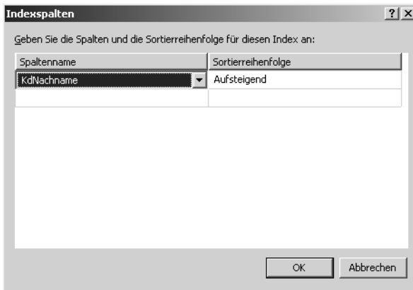
Abbildung 3.29: Indexspalten auswählen
