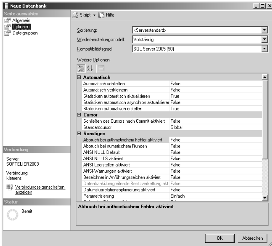
Abbildung 3.9: Datenbankoptionen einstellen
