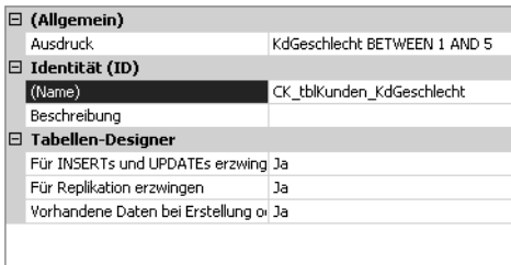
Abbildung 3.21: Einschränkungsname festlegen
