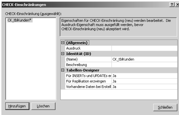
Abbildung 3.19: Neue Check-Einschränkung
