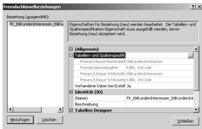
Abbildung 3.25: Neue Fremdschlüsselbeziehung
