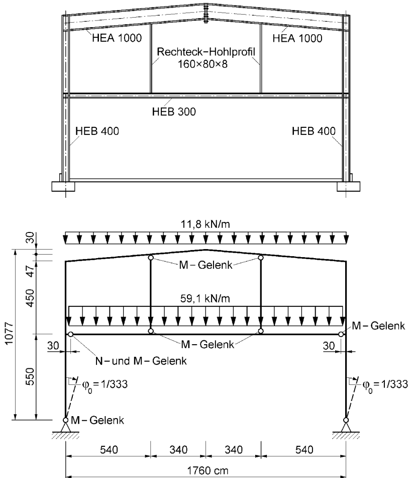
Bild 5.29 Zweigeltenrahmen mit Zwischenbühne
