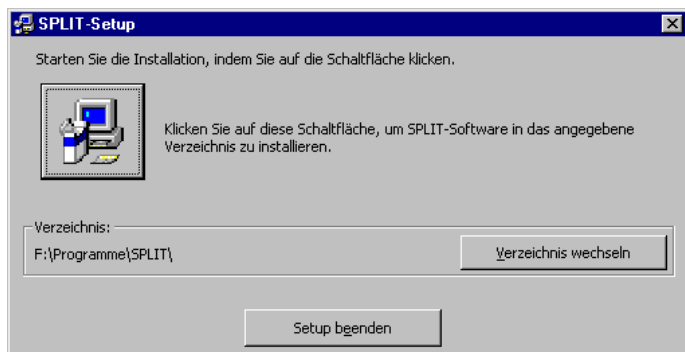
Bild 3.9: Das Setup-Programm
