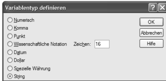
Abbildung 1.8: Datentyp STRING für eine Textvariable mit maximaler Länge von 16 Zeichen
