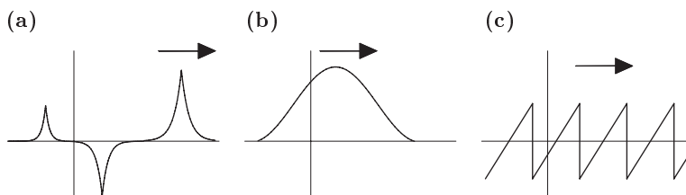
Abb. 6.9. Diverse Wellenformen
