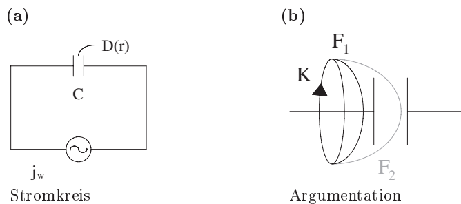
Abb. 6.5. Maxwells Verschiebungsstrom
