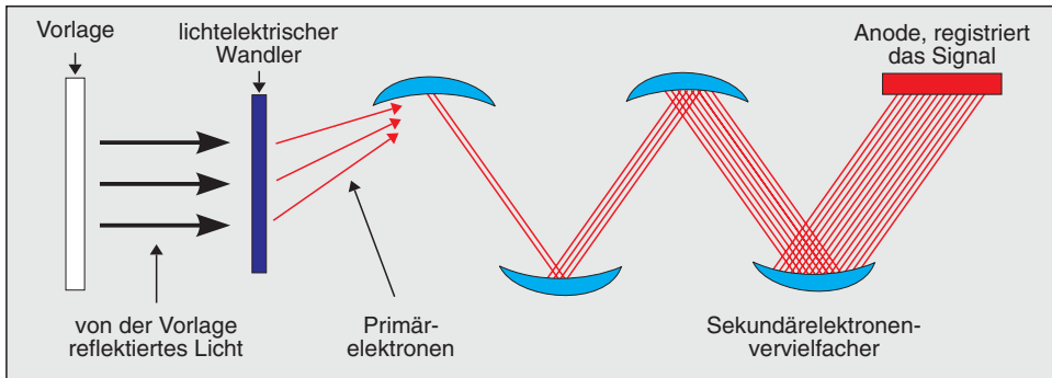
Abbildung 3.7: Funktionsprinzip eines Fotomultipliers
