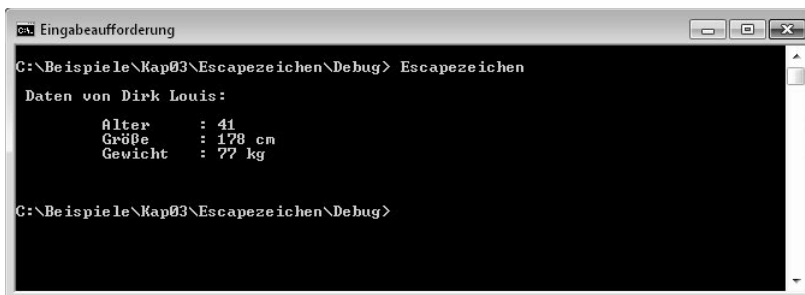
Abb. 3.4: Mithilfe von Tabulatoren, Leerzeichen und Umbrüchen formatierte Ausgabe
