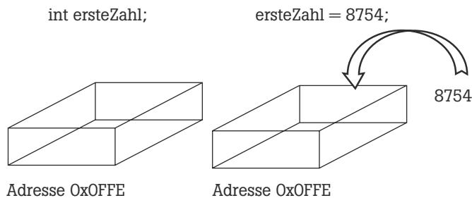
Abb. 3.8: Instanzbildung
