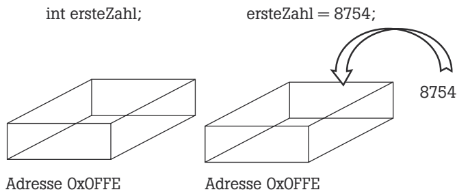
Abb. 3.3: Definition und Zuweisung
